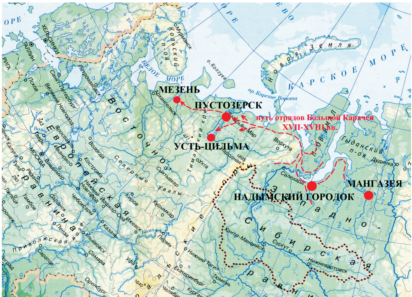
Рис. 1. Карта-схема расположения исторических поселений XVII–XVIII вв.: города Пустозерска, Надымского городка и реконструируемых маршрутов «воровских» операций Большой Карачей в Пустозерском уезде
